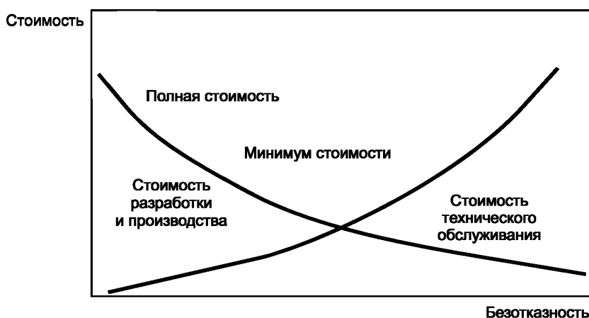
Рисунок 1 — Зависимость стоимости от безотказности
