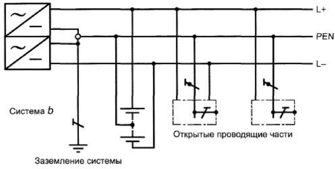
Рисунок 31G - Система TN-C постоянного тока
