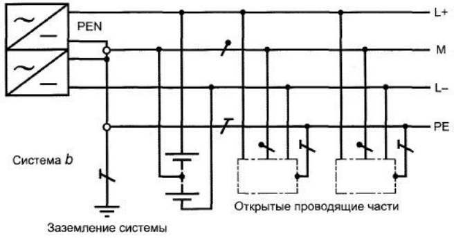
Рисунок 31F - Система TN-S постоянного тока
