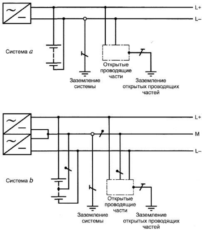
Рисунок 31J - Система TT постоянного тока
