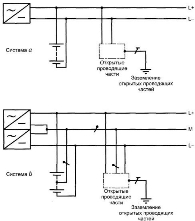
Рисунок 31К - Система IT постоянного тока
