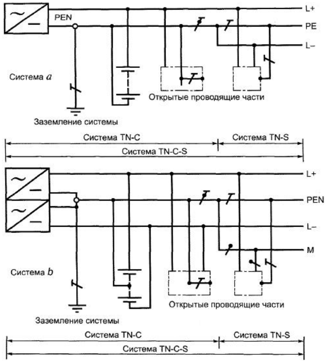
Рисунок 31H - Система TN-C-S постоянного тока
