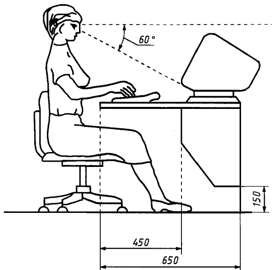
Рисунок 1. Расположение дисплея на столе
